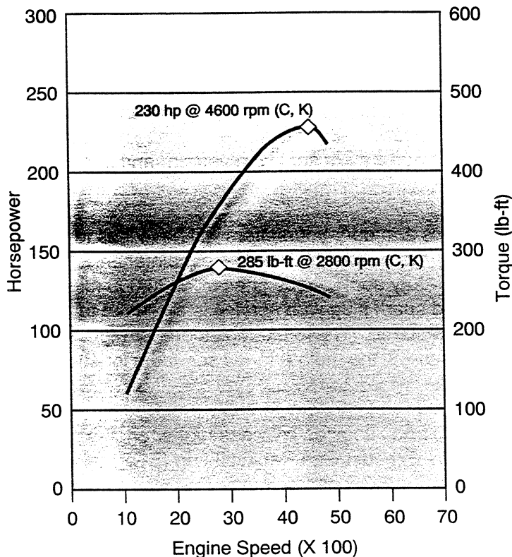
"Vortec 5000" (L30)
