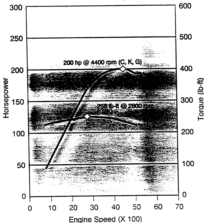
"Vortec 4300" (L35)
