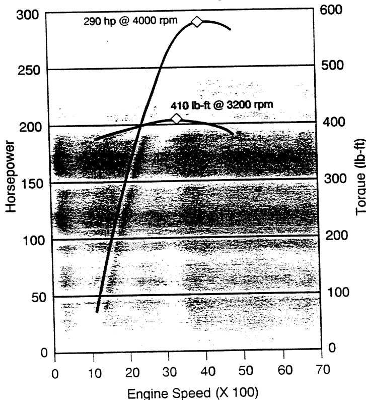
"Vortec 7400" (L29)
